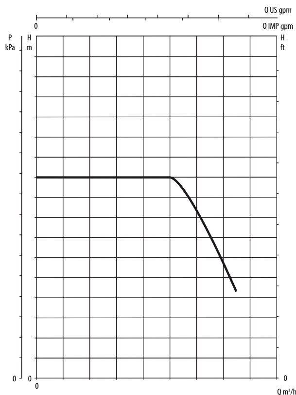
Рис. 7 Гидравлические характеристики насоса с использованием инвертора
