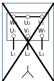
3 Неправильное подключение
