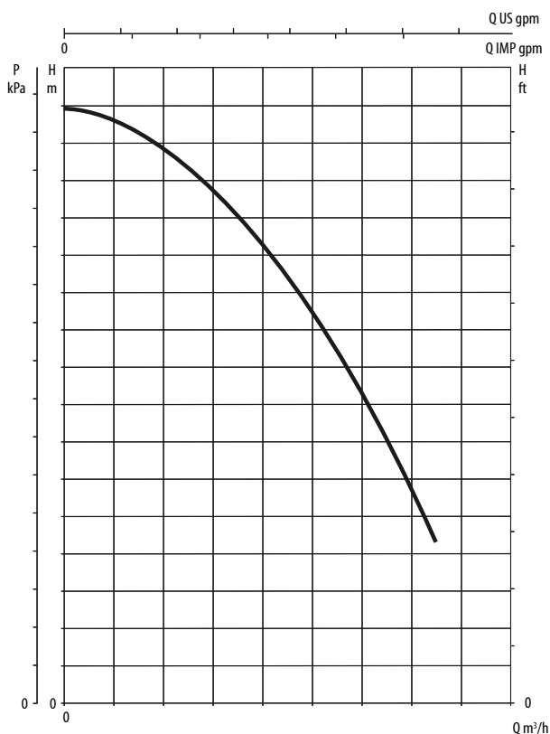
Рис. 6 Гидравлические характеристики насоса без использования инвертора
