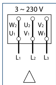
4 Правильное подключение
